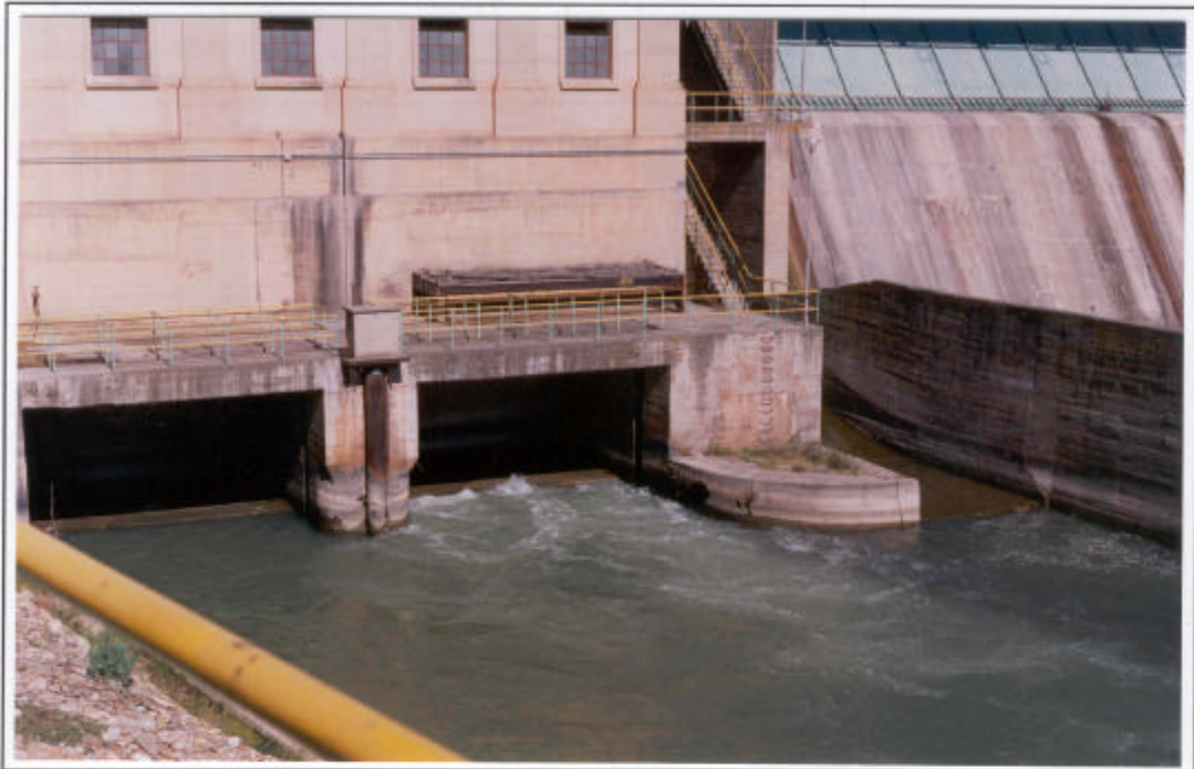
Compuertas de fondo de la presa de San Lorenzo Mongay.
